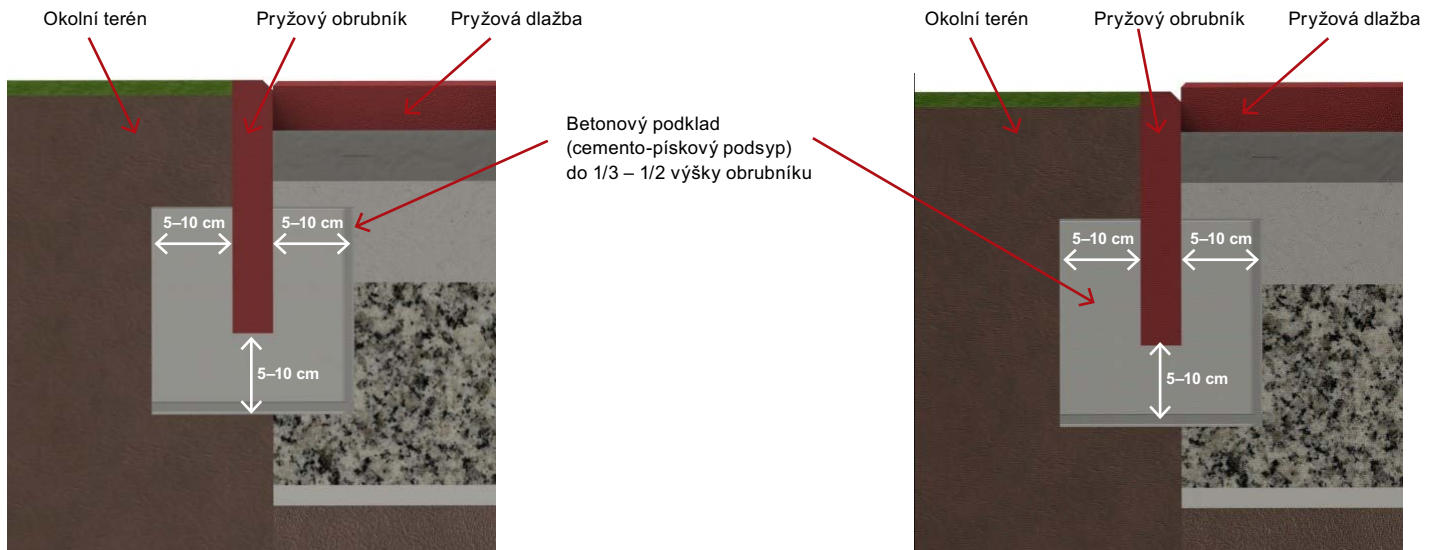
Obr. 01: Standardní použití pryžového obrubníku
